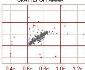
СКАТТЕРОГРАММА
